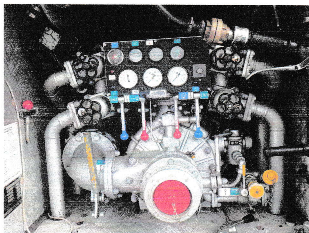
Fot. 9. Autopompa.
